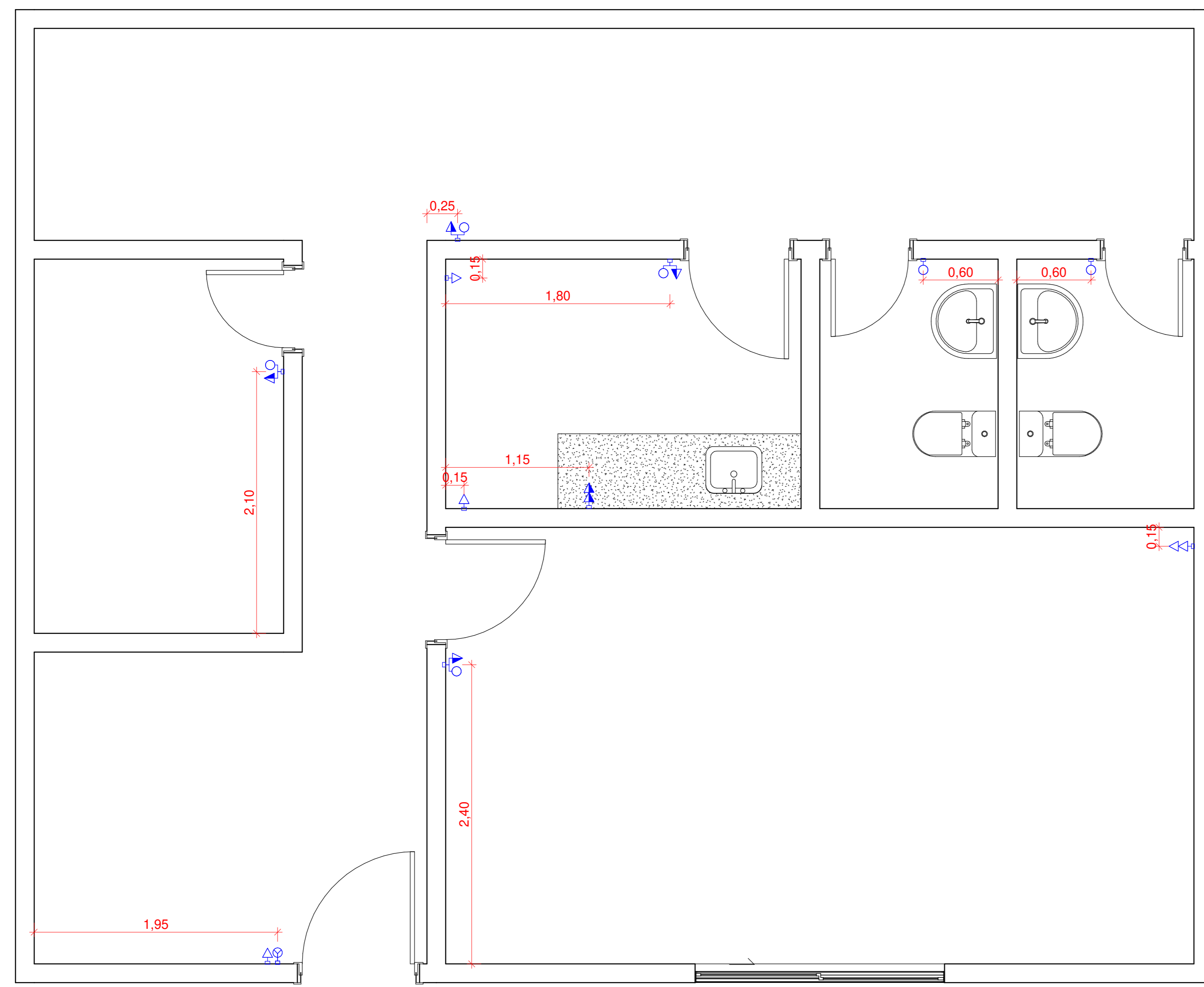
4 PONTOS ELETR._HIDRO 1 : 25
