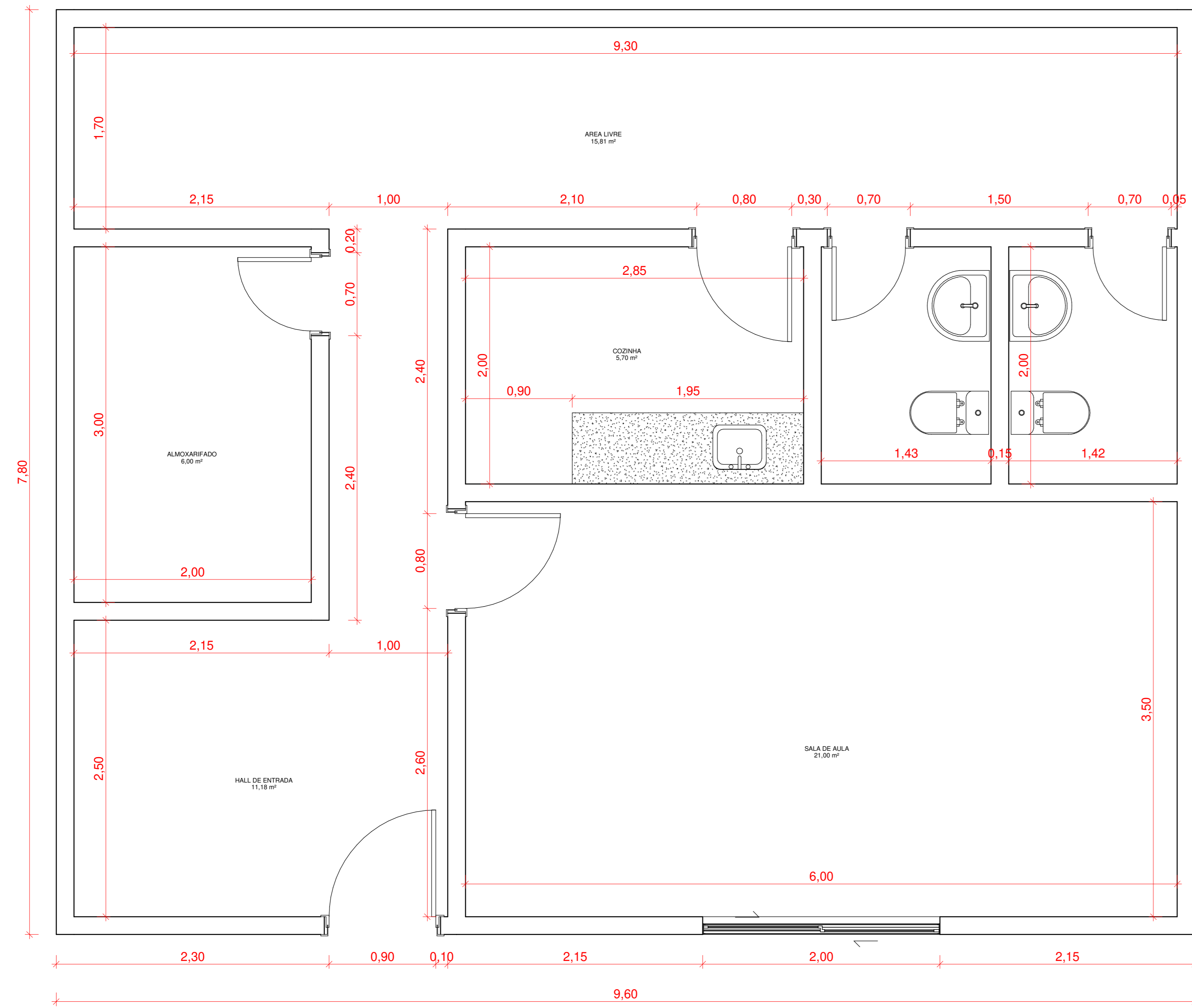
1 PLANTA BAIXA 1 : 25
